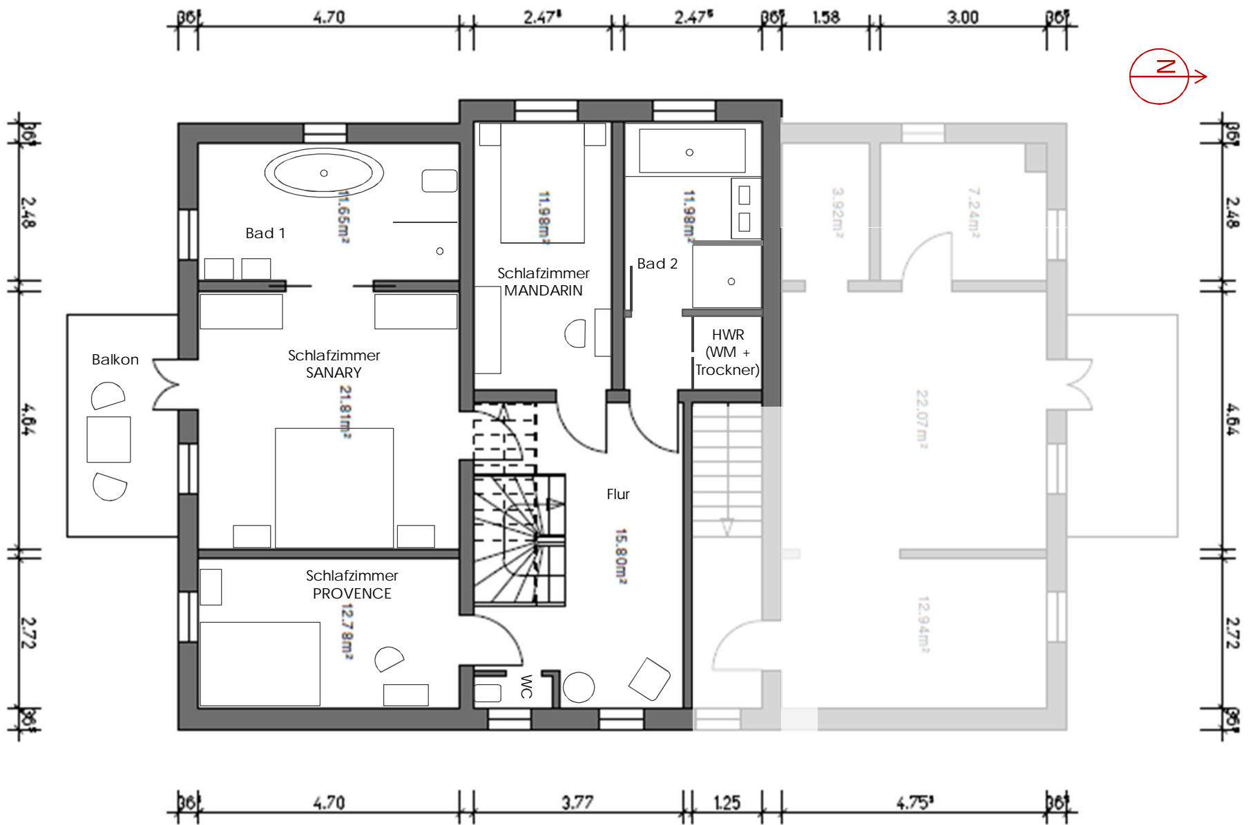
VILLA FRANCA - Grundriss 1. Obergeschoss
